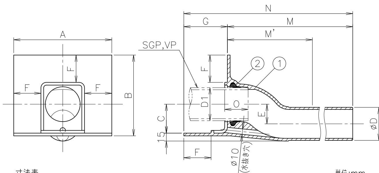
寸法表
