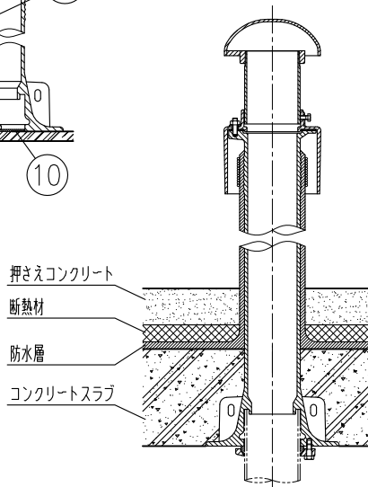
施工例
