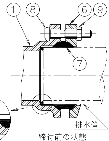
継手各部の名称 締付後の状態
