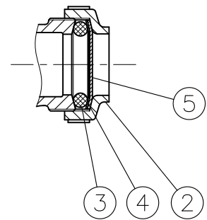
出荷時の部品構成
