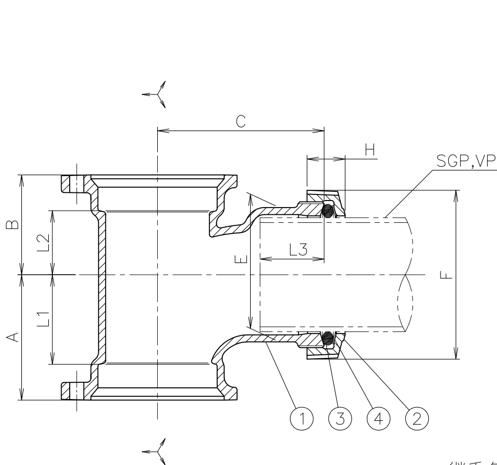
継手各部の名称
