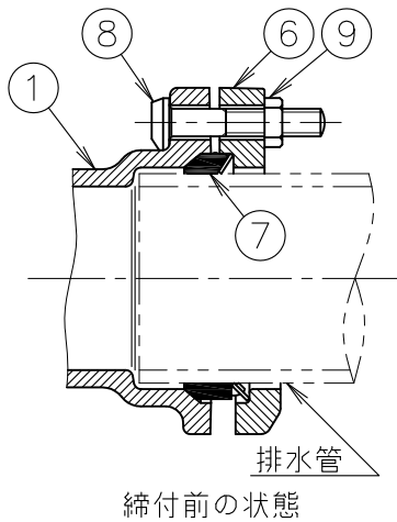
継手各部の名称
