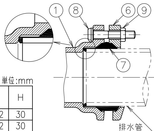
締付前の状態
