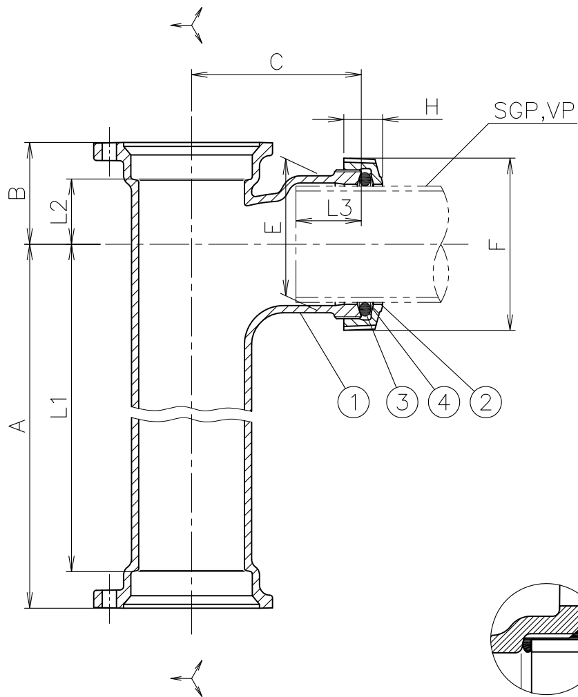
継手各部の名称 締付後の状態
