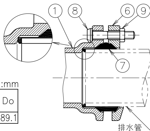
継手各部の名称 締付後の状態
