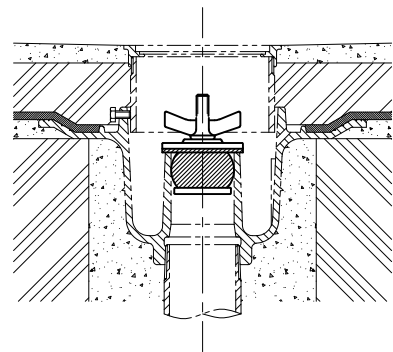
満水テストプラグ設置例 <呼び 45・50>
