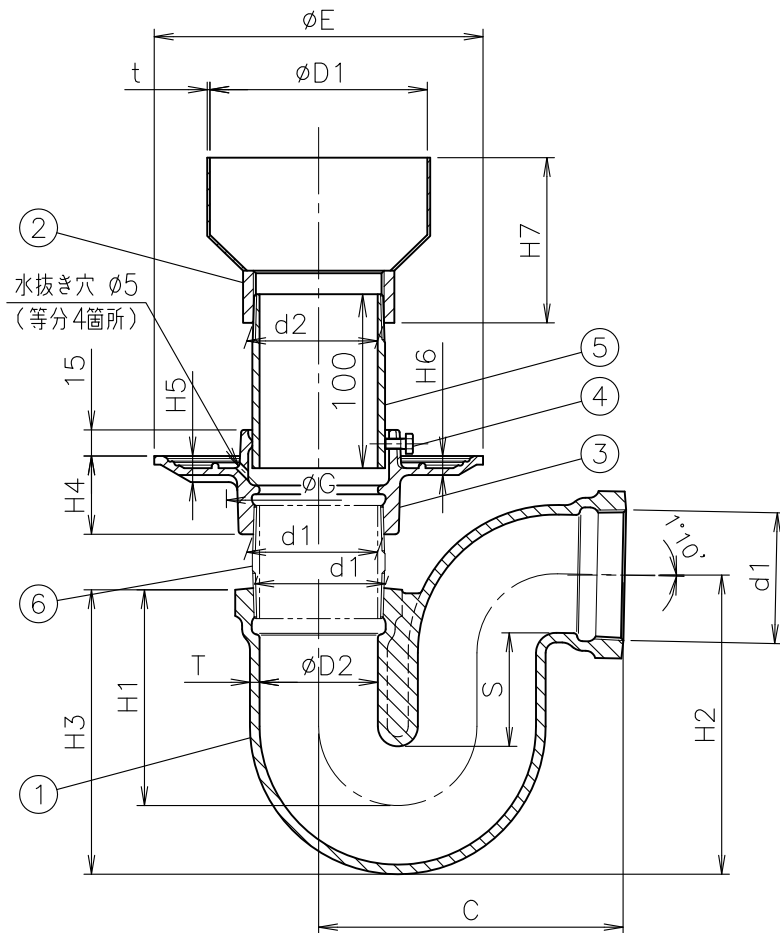
寸法表
