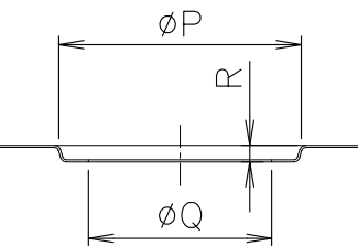
金属流し台トラップ取付 加工寸法表
