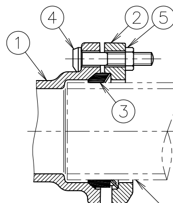
継手各部の名称
