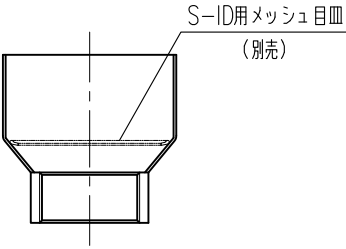
S-ID用メッシュ目皿設置図(2:3)
