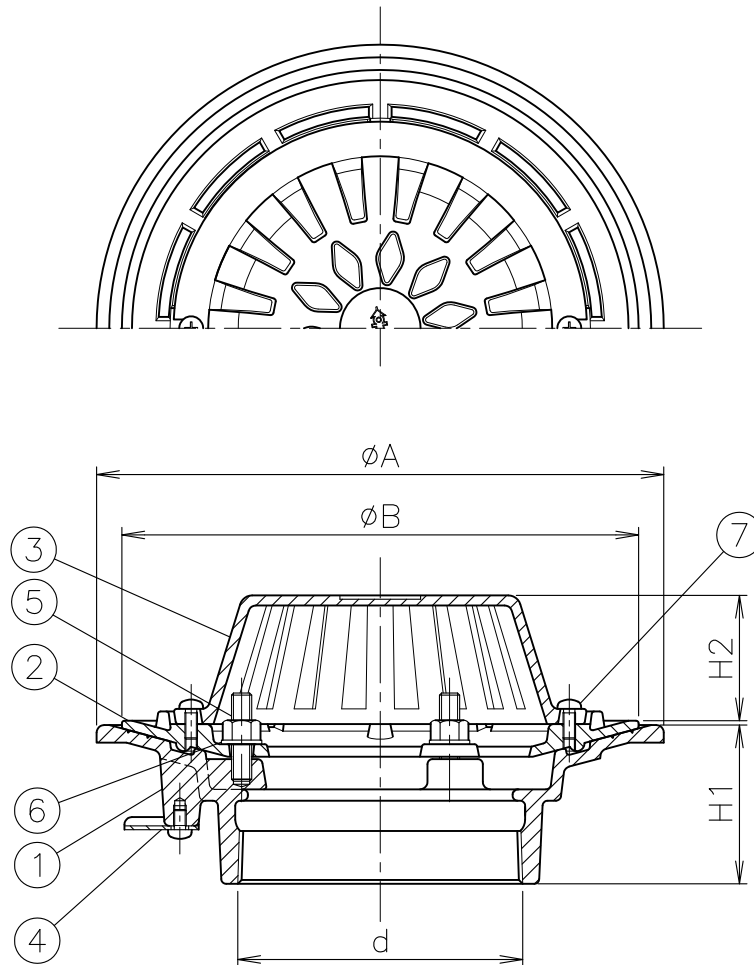
寸法表
