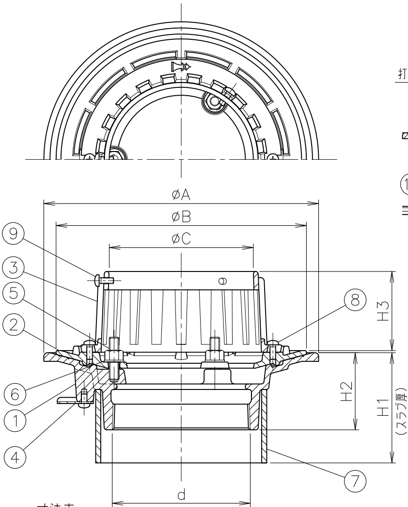
寸法表
