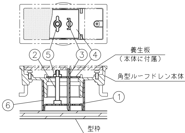
打込金具 固定図(1:4)
