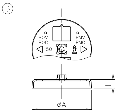
寸法表
