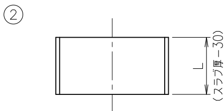
寸法表
