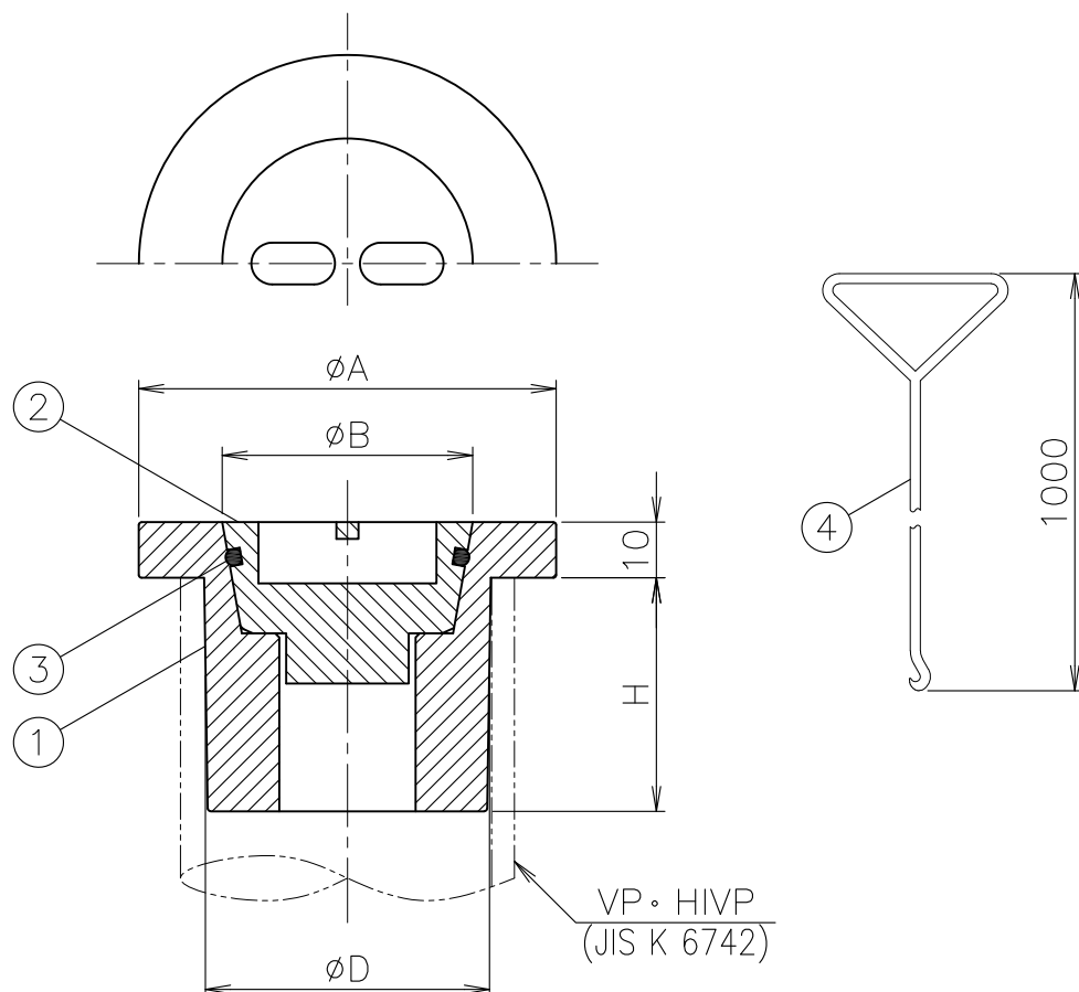
寸法表
