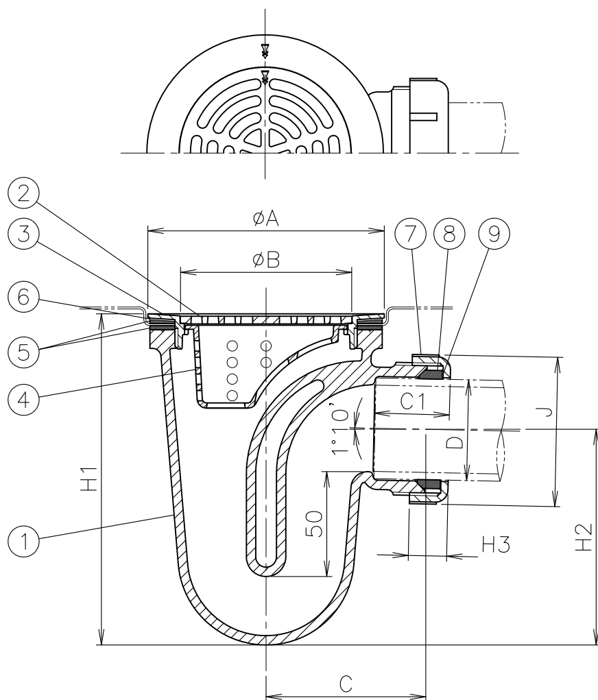
寸法表
