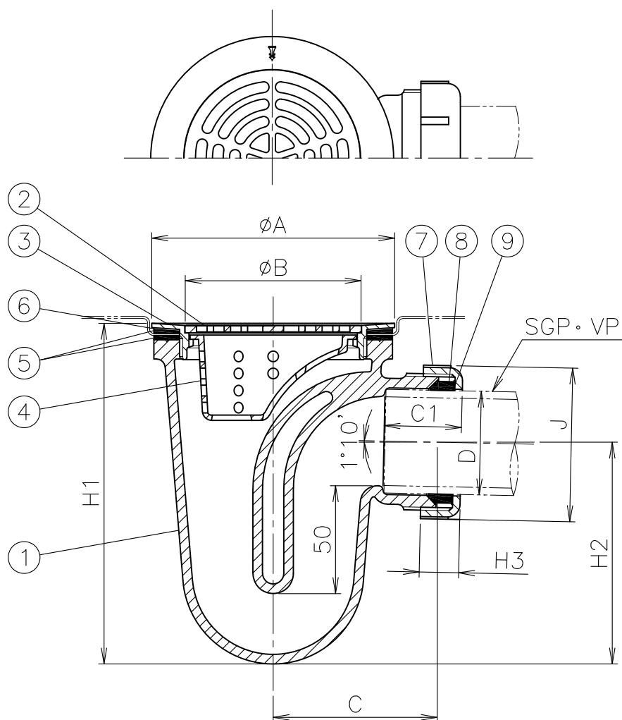
寸法表
