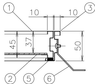
端部詳細
