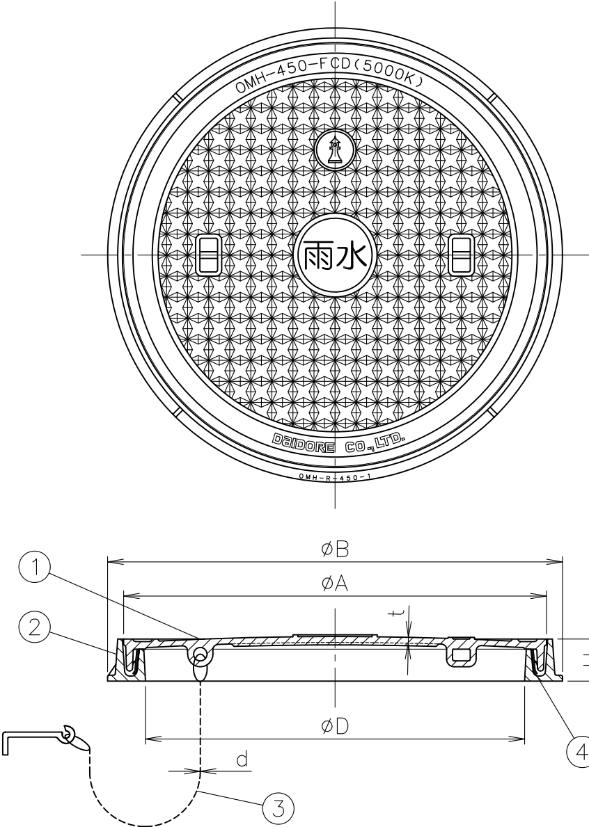
端部詳細
