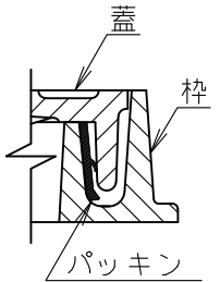
端部詳細
