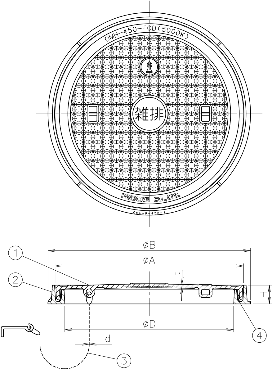
端部詳細
