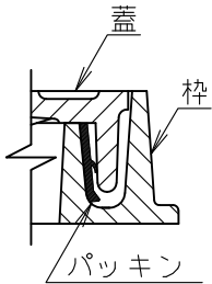
端部詳細
