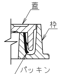
端部詳細
