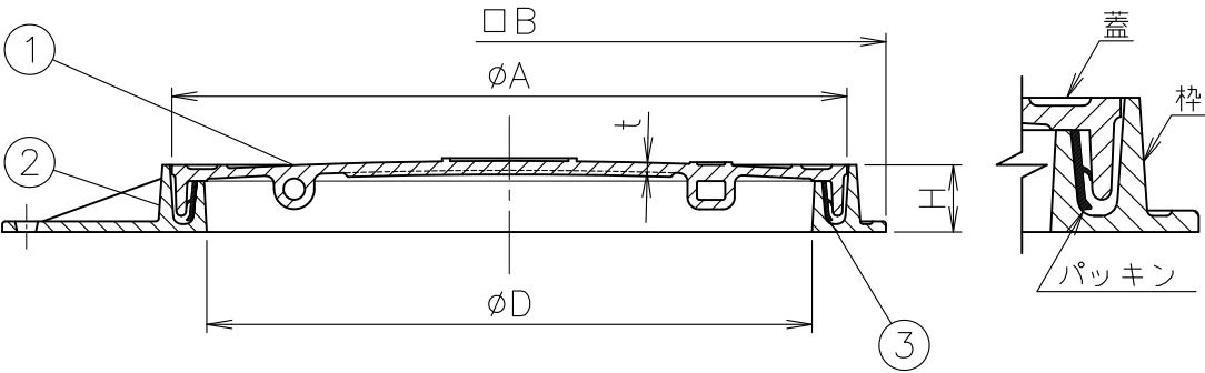
端部詳細
