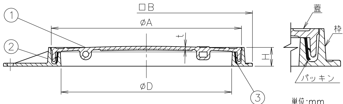
端部詳細
