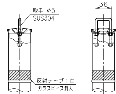
頭部取手詳細図 (3:1)
