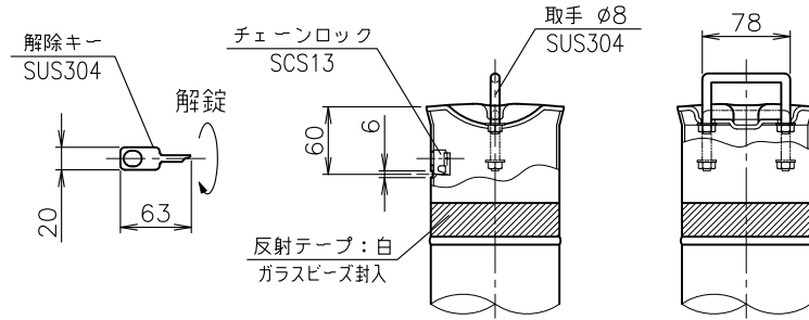
頭部取手詳細図(2:1)
