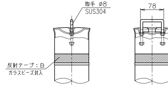
頭部取手詳細図(2:1)
