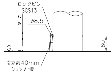
地祭部詳細図(2:1)
