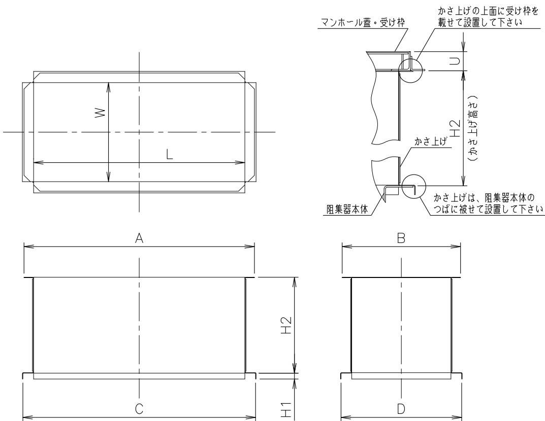
寸法表
