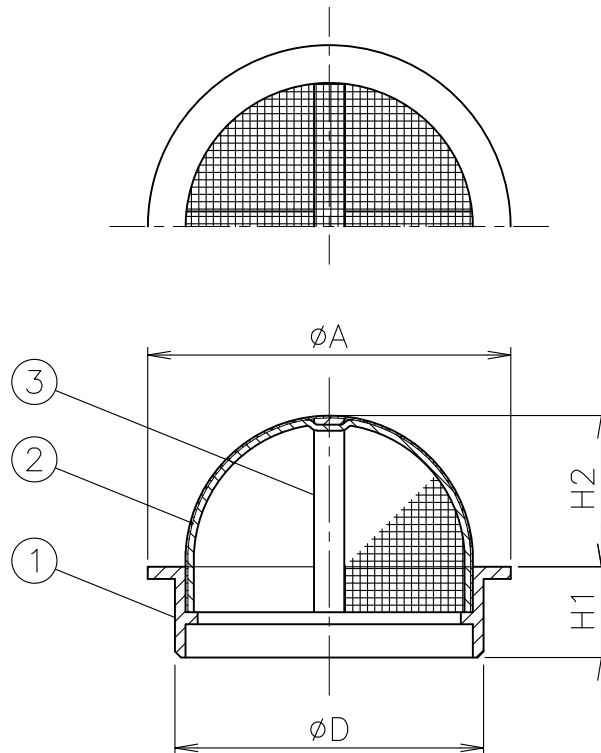
寸法表
