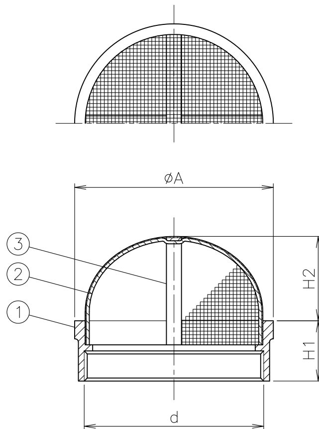
寸法表
