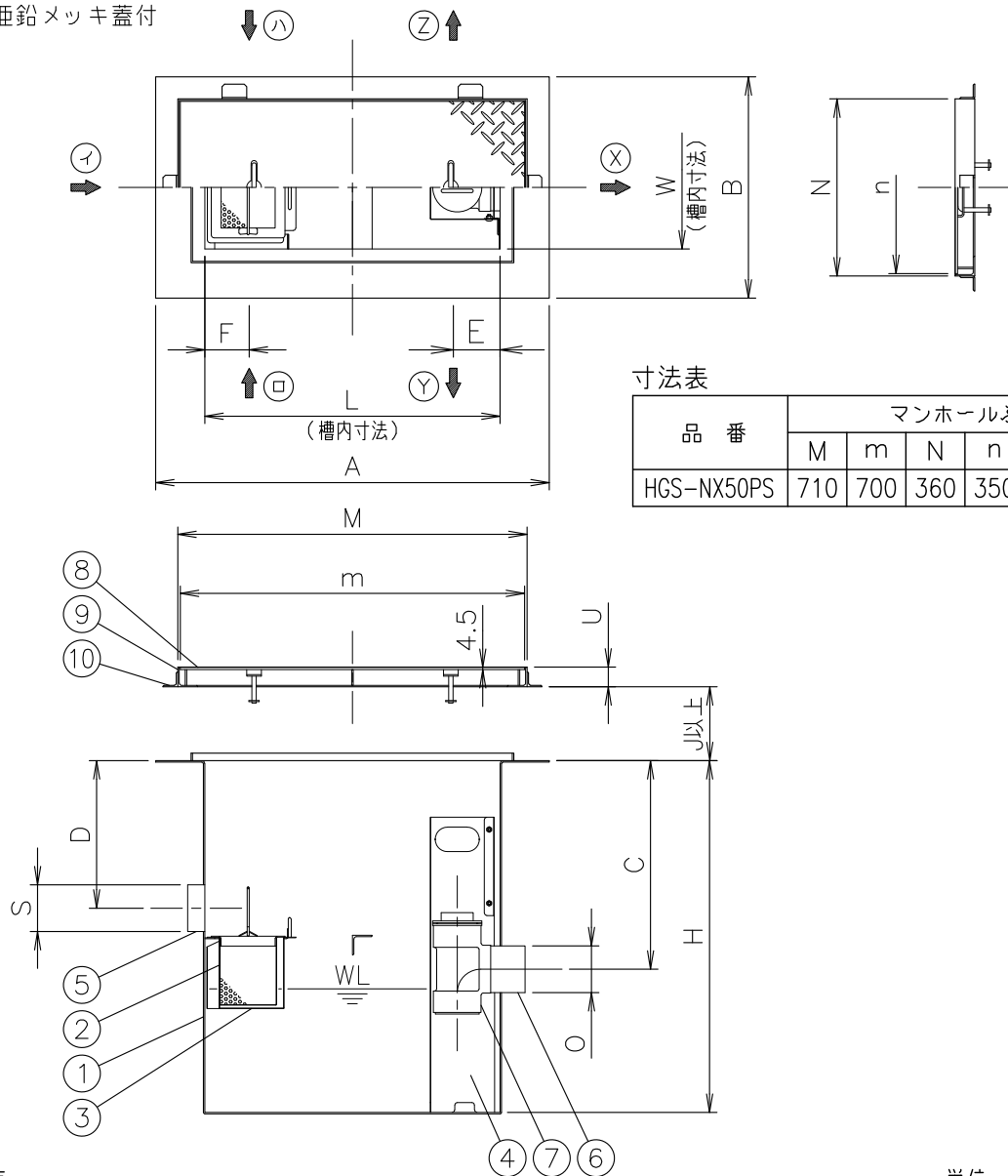
寸法表 単位:mm
