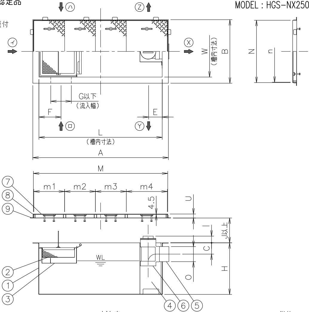
寸法表
