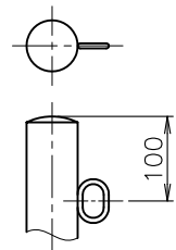
片フック (F01)
