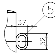
フック部詳細図(2:1)
