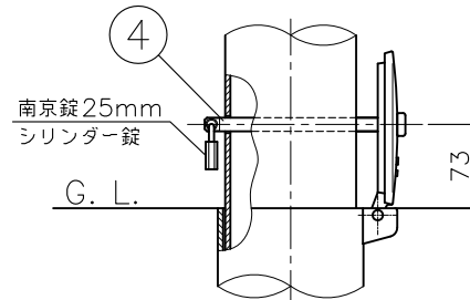
施錠部詳細図 (2:1)
