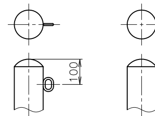
片フック (F01)
