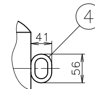
フック部詳細図 (2:1)
