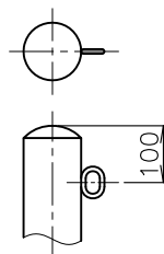
片フック (F01)
