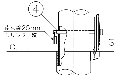
施錠部詳細図 (2:1)
