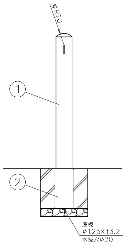
片フック (F01)
