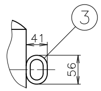
フック部詳細図 (2:1)
