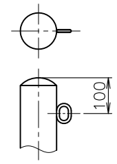
片フック (F01)
