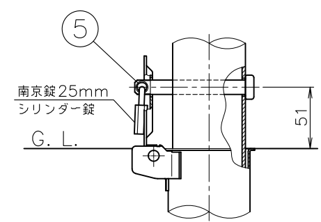
施錠部詳細図(3:1)
