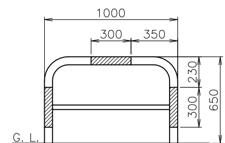
塗装色(赤・白/緑・白)配色図(1:2)
