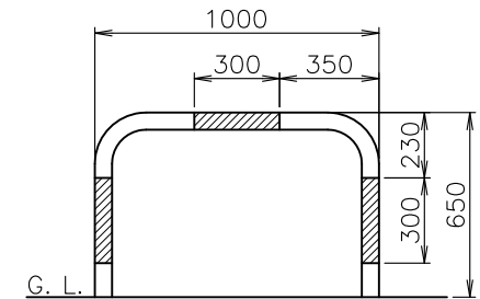
塗装色(赤・白/緑・白)配色図(1:2)
