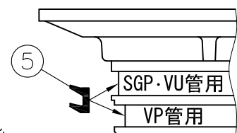
パッキン取り付け位置
