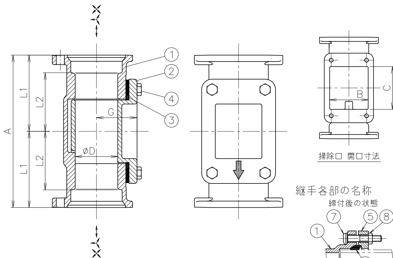
寸法表
