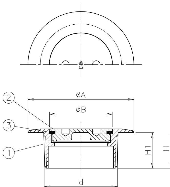
寸法表
