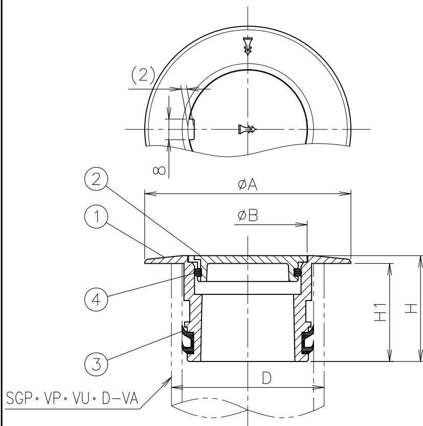
寸法表
