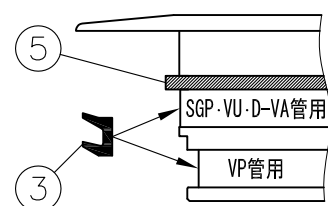
パッキン取り付け位置
