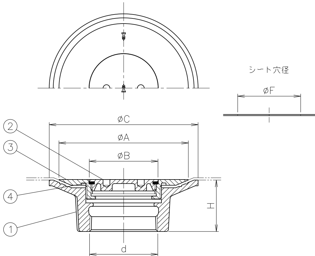
寸法表 単位:mm
