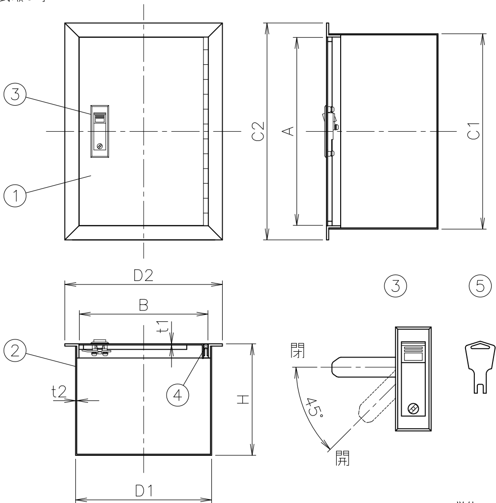
寸法表 単位:mm
