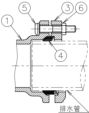
締付前の状態
