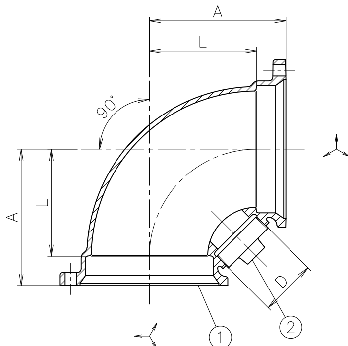
継手各部の名称 締付後の状態
